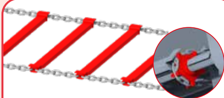
Listwy rurowe przyspawane do łańcuchów ogniowych 14 (zapobieganie osadzaniu się materiału) + zębátky spawane.
